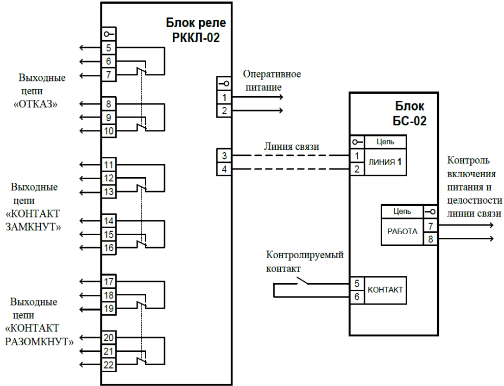
Схема подключения блока реле РККЛ-02 и блока БС-02
