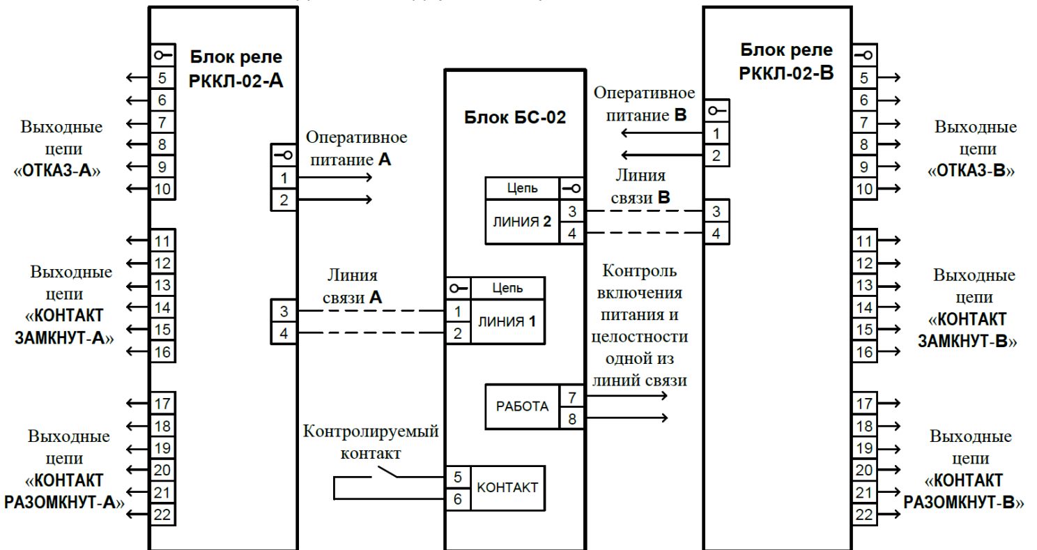
Схема подключения двух блоков реле РККЛ-02 и блока БС-02
