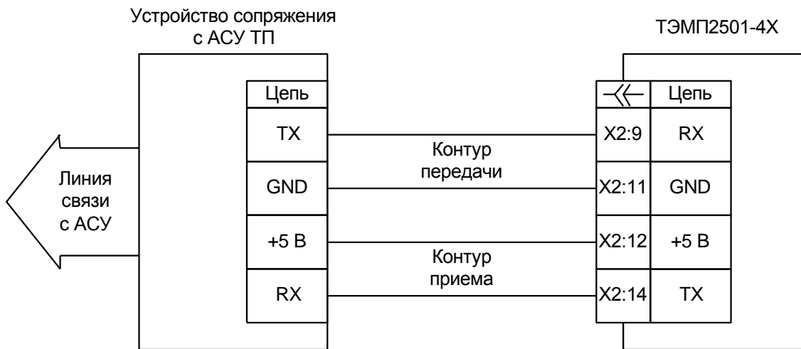
Рисунок В.3 – Схема подключения устройства ТЭМП 2501-4X исполнения TTL к отдельному каналу связи устройства сопряжения с АСУ ТП
