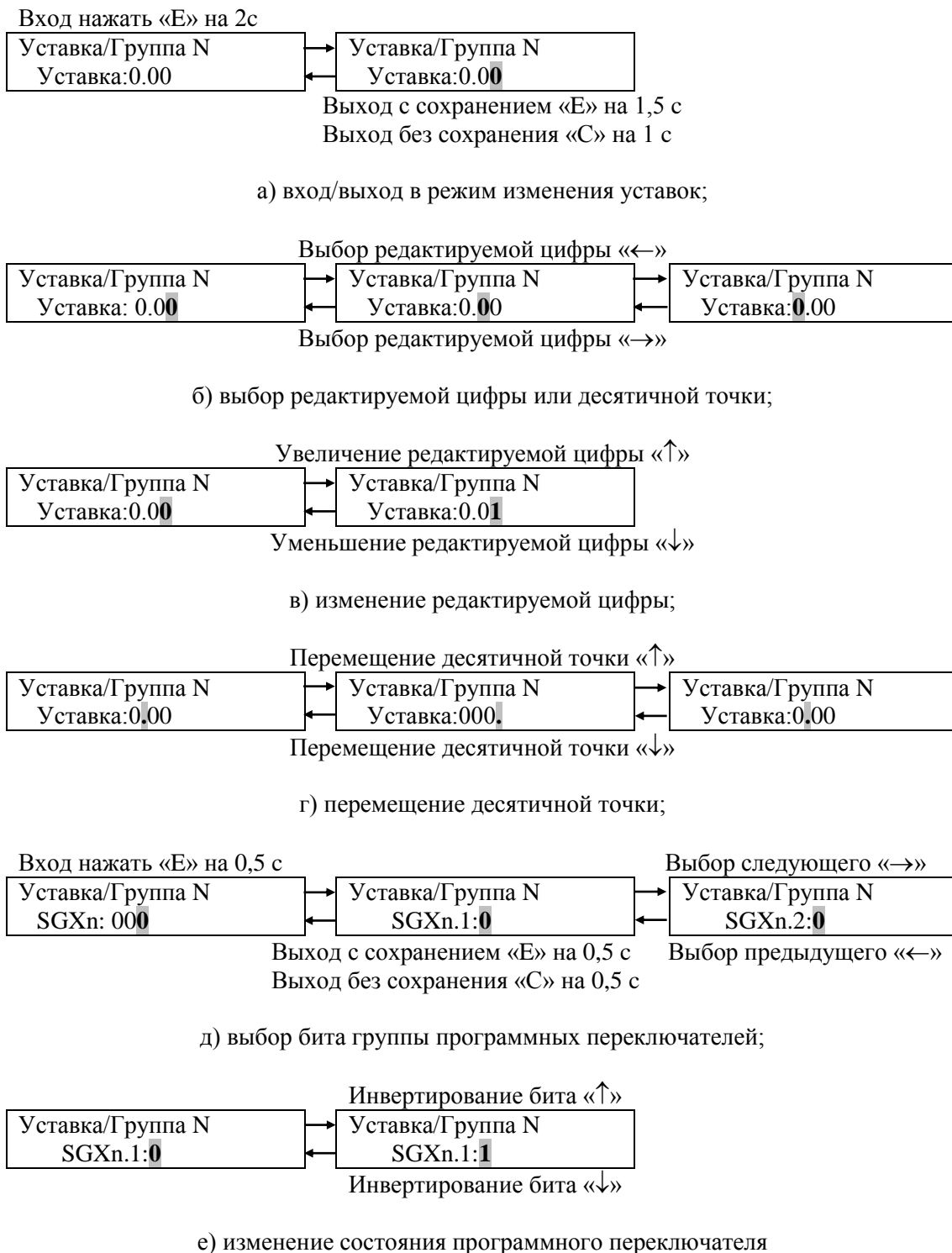
Рисунок 2.2 - Действия, осуществляемые кнопками при редактировании уставок/параметров устройства
