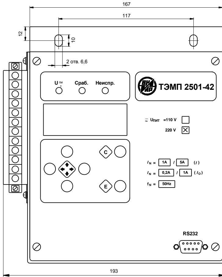
Рисунок А.5 – Вид спереди ТЭМП 2501-42
