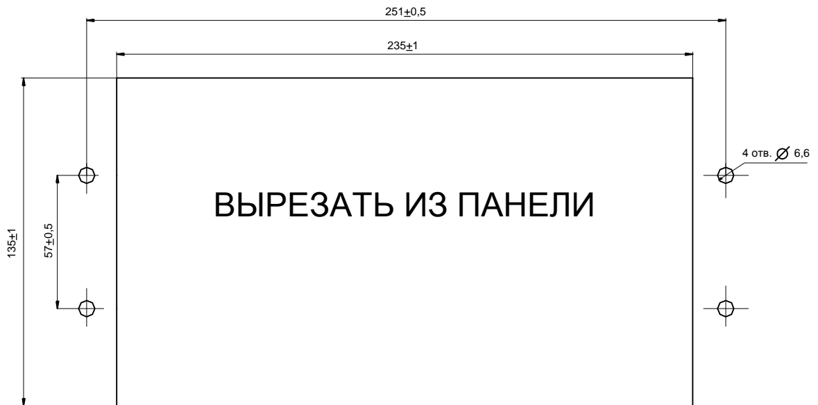
Рисунок А.4 – Установочные размеры ТЭМП 2501-41
